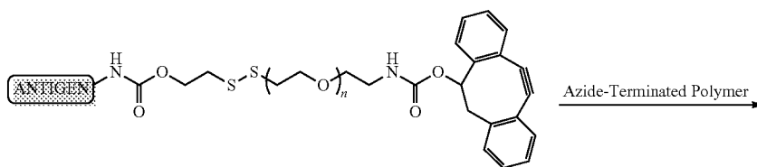
DIBO-PEG2K-Amine-Antigen Conjugate
