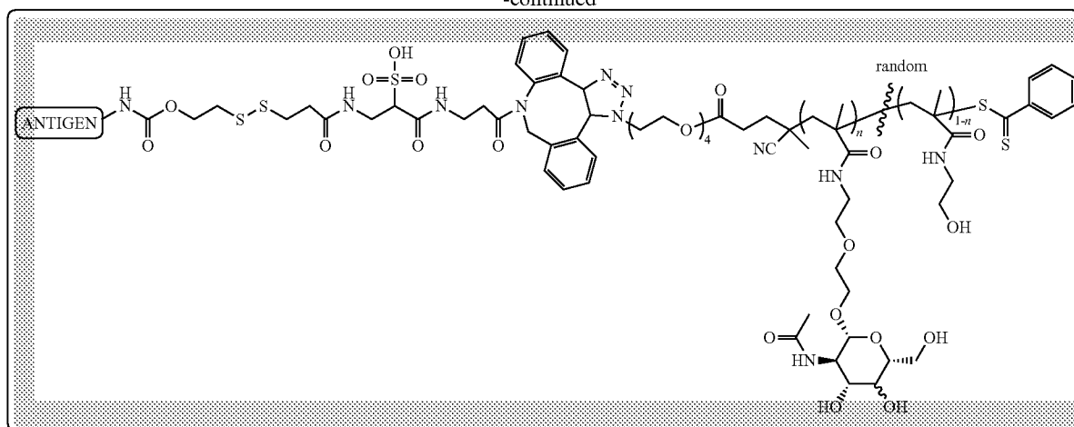
Antigen-NH-(S-DBCO)-P(GalNAc-co-HEMA) Conjugate -OR- Antigen-NH-(S-DBCO)-P(GlcNAc-co-HEMA) Conjugate
