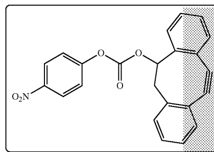
DIBO-NPC
