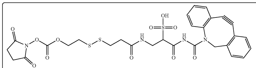
S-DBCO-NHS
