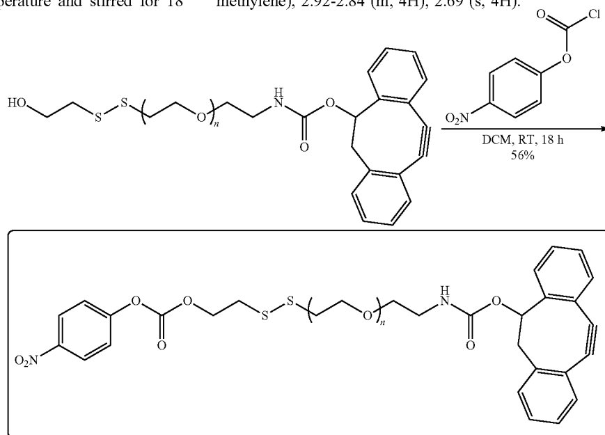
DIBO-PEG2K-NPC
