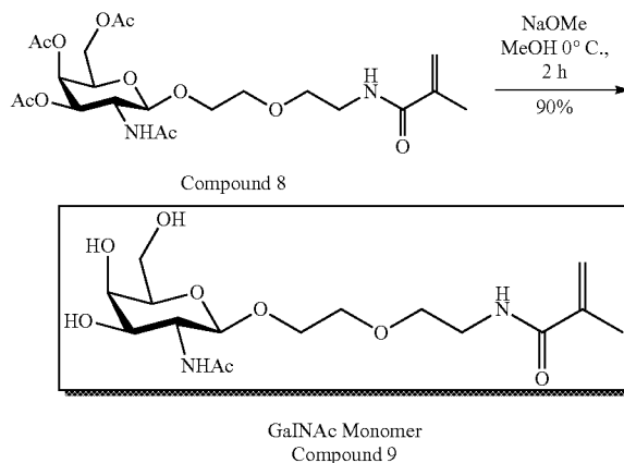
GalNAc Monomer (9)
