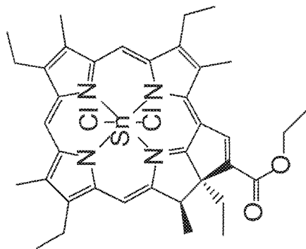
Rostaporfin (Purlytin)
