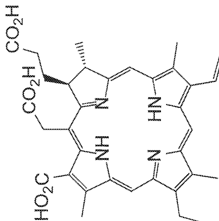
Chlorin e6
