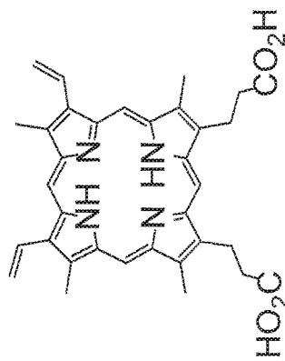
Protoporphyrin IX
