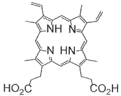
Protoporphyrin IX
