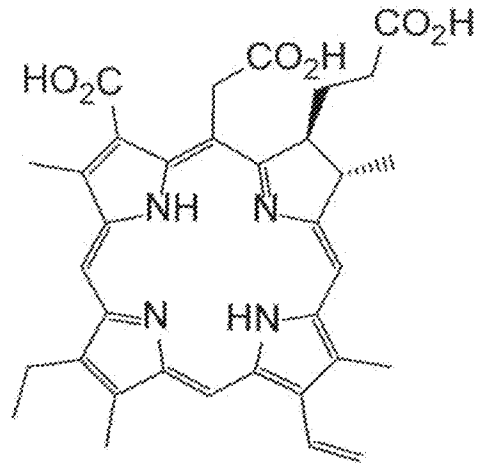
Chlorin e6
