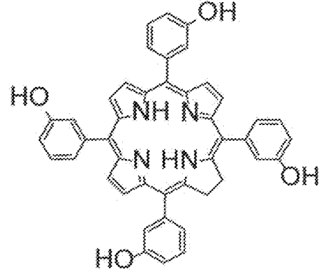
m-THPC (Foscan)
