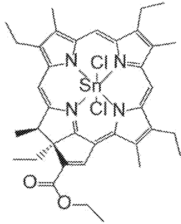
Rostaporfin (Purlytin)
